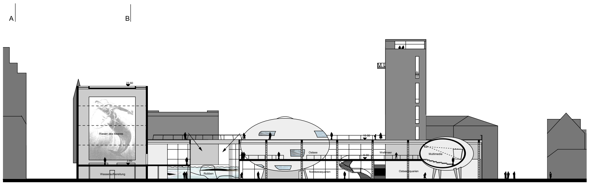
SCHNITT B-B 1:200
